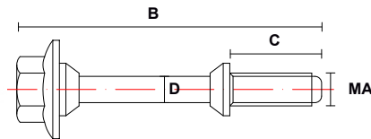
IMG 1 - Perno especial 1
