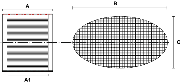
Filtro de partículas ovalado SIC
