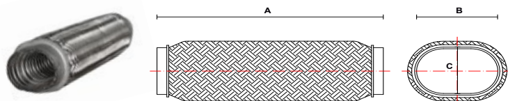
IMG 2 - Tubo flexible interior acanalado ovalado
