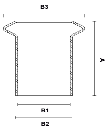
Cono con reborde cónico
