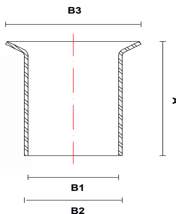
Cono simple
