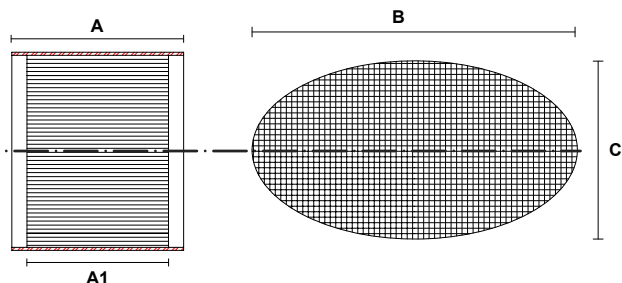
Sustrato Metálico Oval
