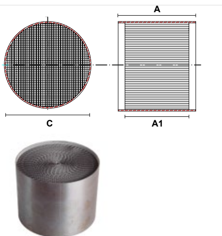
Sustrato Metálico Redondo
